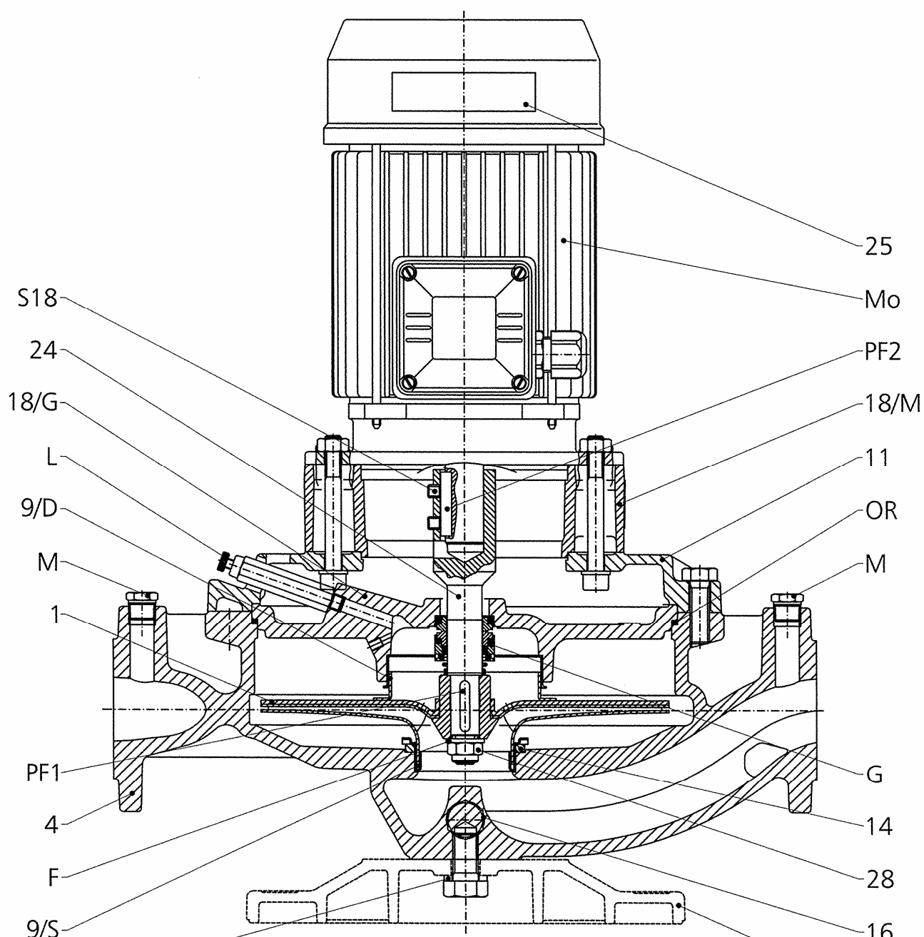
Разрез насоса LR
